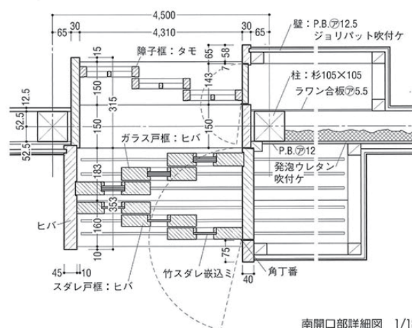
南開口部詳細図 1/18
