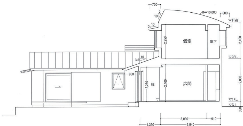
断面図 1/125
