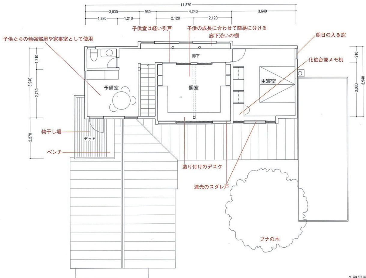
2 階平面図 1/125
